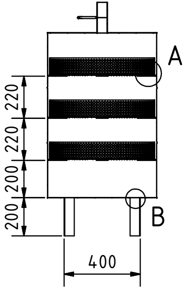
A-A ( 1 :20 )
