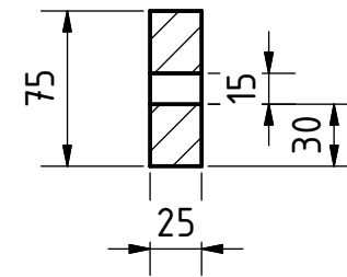
D-D ( 1 : 4 )
