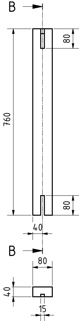
ELEVATION ( 1 : 8 )
