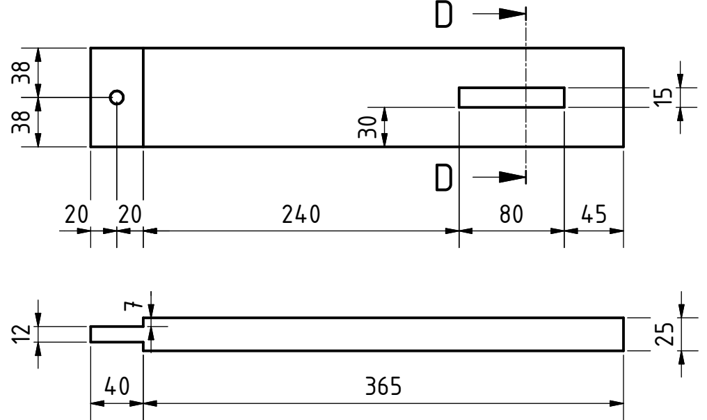
PLAN ( 1 : 4 )
