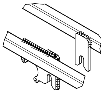
G ( 1 : 5 )
