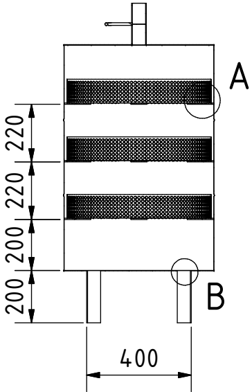
A-A ( 1 :20 )
