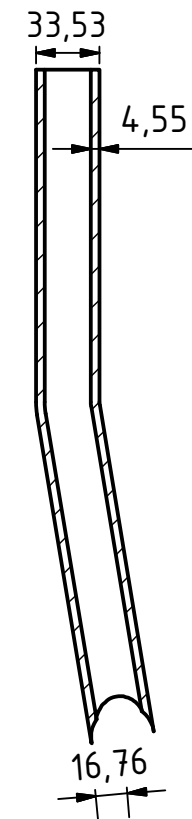
C-C ( 1 : 4 )
