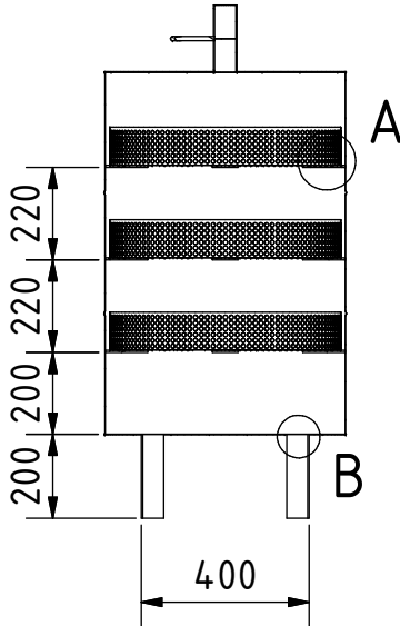
A-A ( 1 :20 )
