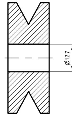
SECTION MD-MD SCALE 1 : 1
