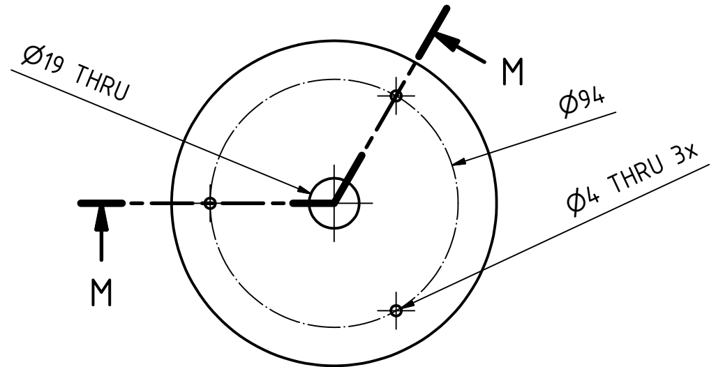
M-M ( 1 : 2 )
