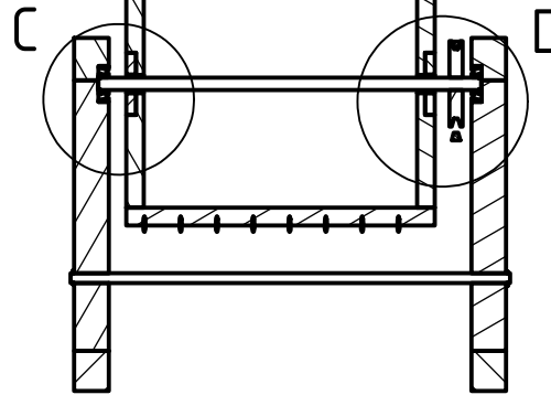
A-A ( 1 : 12 )
