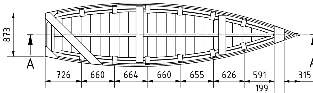
A-A ( 1 : 40 )
