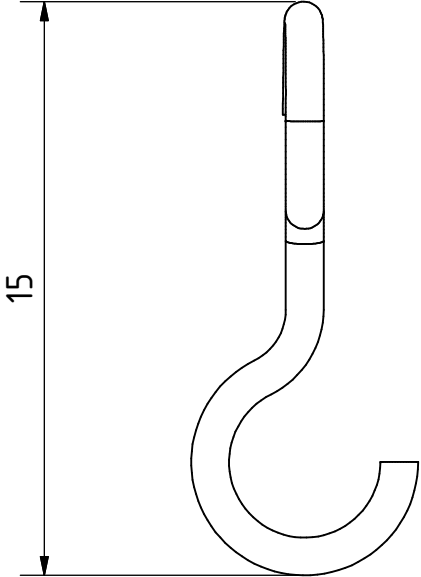
ELEVATION ( 5 : 1 )
