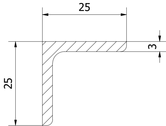
AJ-AJ ( 1.5 : 1 )
