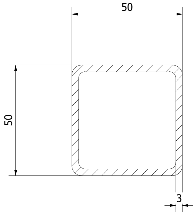
AM-AM ( 1 : 1 )
