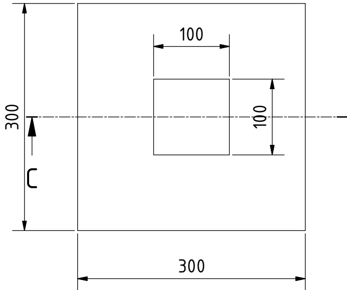
PLAN ( 1 : 5 )
