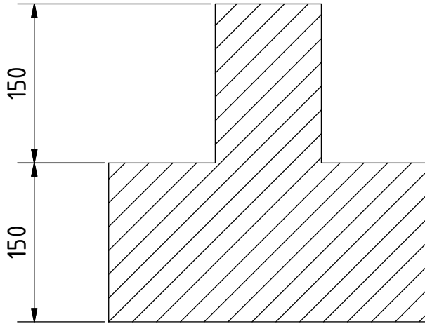
C-C ( 1 : 5 )
