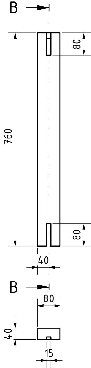
ELEVATION ( 1 : 8 )
