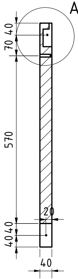
B-B ( 1 : 8 )
