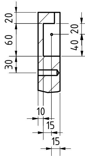
A ( 1 : 4 )
