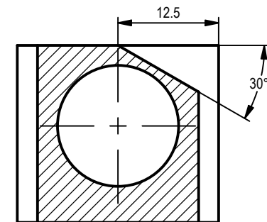
SECTION MG-MG SCALE 1.5 : 1
