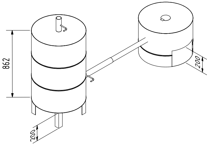
A ( 1 : 5 )
