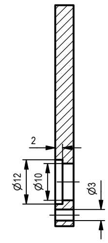
SECTION MG-MG SCALE 1 : 1
