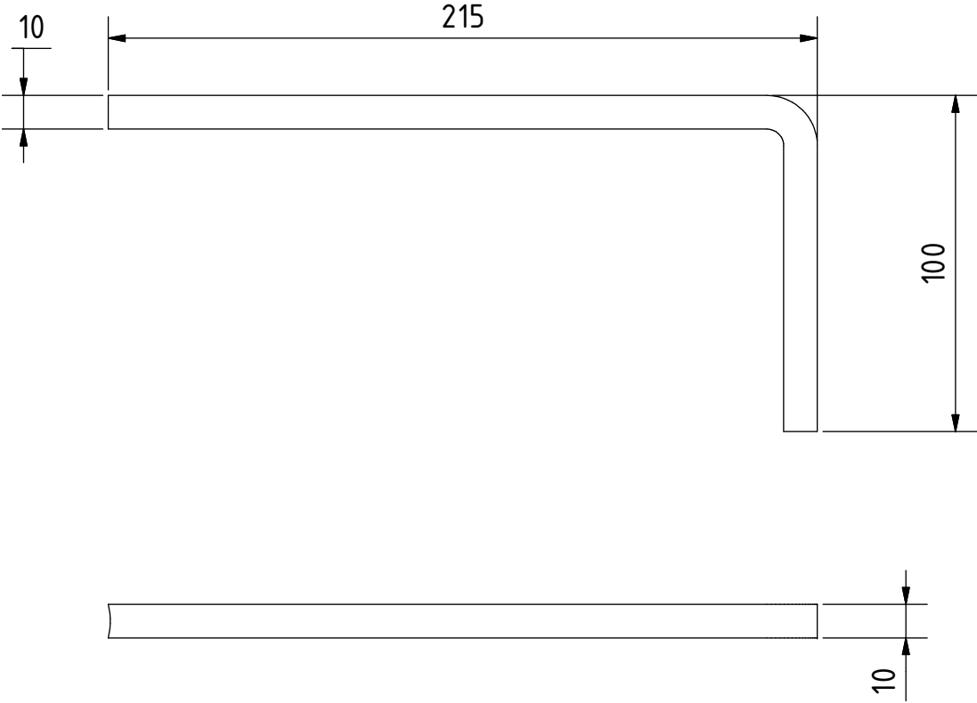
PLAN ( 1 : 2 )
