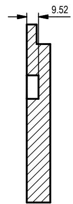
SECTION ME-ME SCALE 1 / 3
